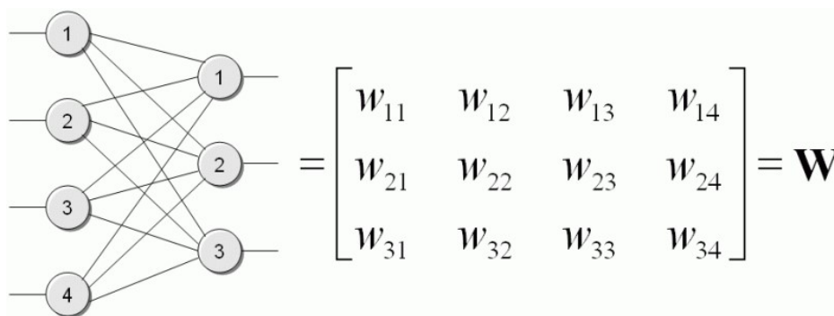
Abbildung 12: Gewichtsmatrix eines neuronalen Netzes (NN7)
